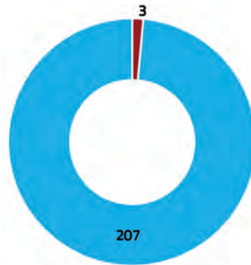
Physik-Nobelpreis
